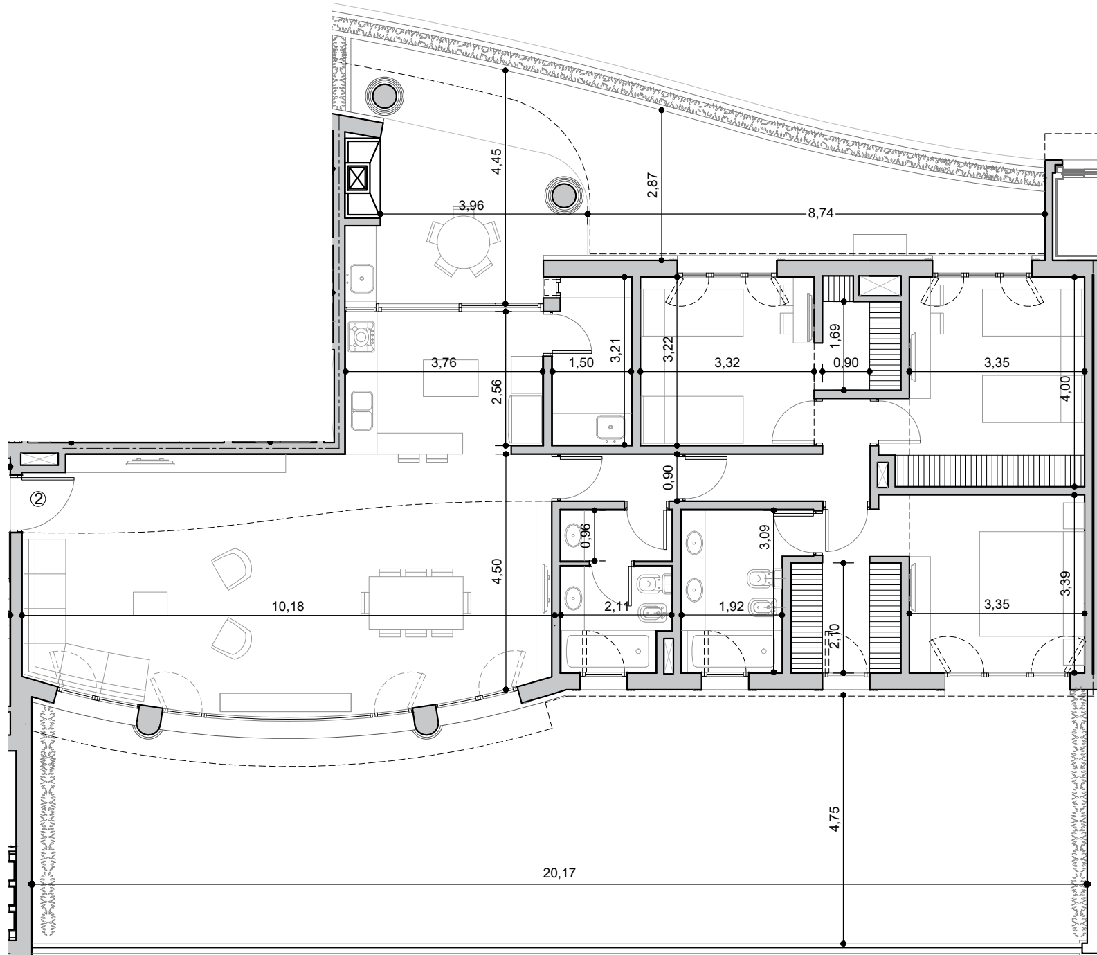
ATENEA 2 Escala 1.100
